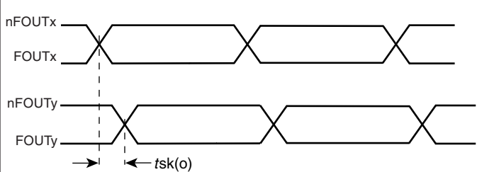
OUTPUT SKEW
