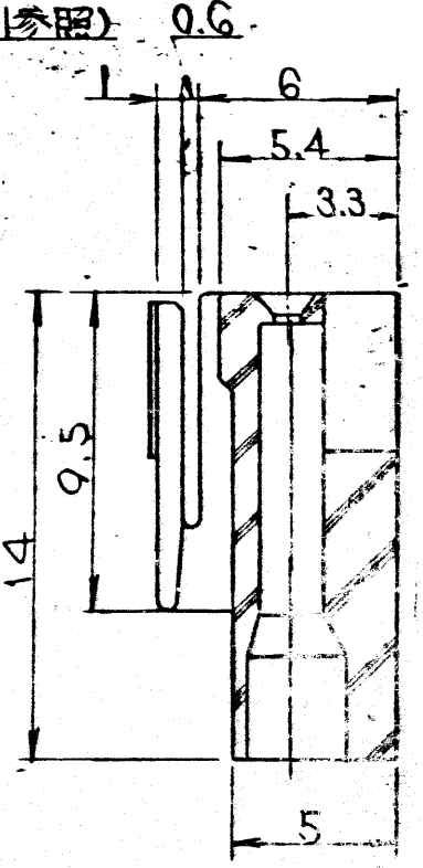
A-A断面図
