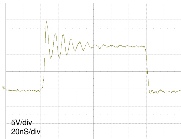
Vsw of iP2003A
