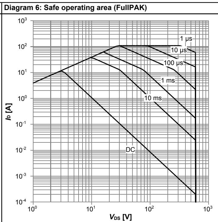
I_D=f(V_{DS}); T_C=25\text{ }^\circ\text{C}; D=0; \text{parameter: } t_p
