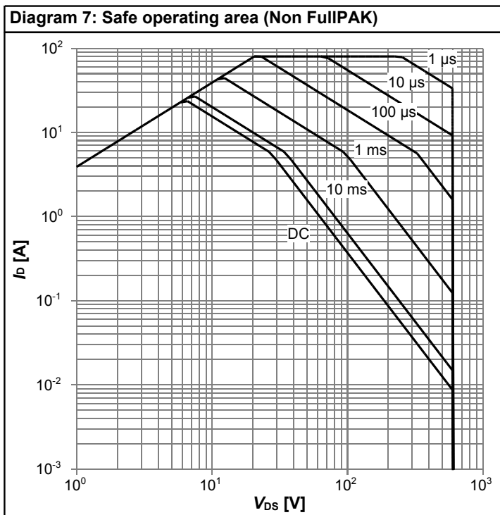
I_D=f(V_{DS}); T_C=80\text{ }^\circ\text{C}; D=0; \text{parameter: } t_p
