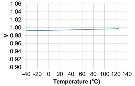
EN_UVLO_STOP
