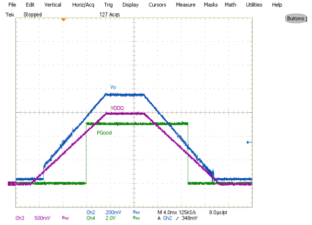
Fig. 14: Tracking -3A load, sinking current, Ch 2 : V_{out} , Ch 3 : I_L , Ch 3 : V_{DDQ} , Ch 4 :PGood
