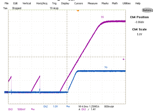
Fig. 12: Short (Hiccup) Recovery Ch 1 : V_{out} , Ch 3 : V_{SS}
