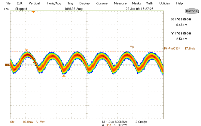
Fig. 20. Output Voltage Ripple, 4A load Ch 1 :V o
