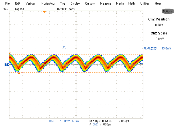
Fig. 20. Output Voltage Ripple, 4A load Ch 2 :V o
