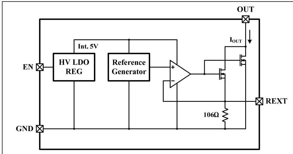
IS31LT3172
