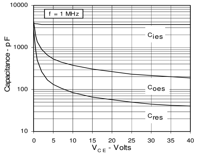
Fig. 16. Capacitance
