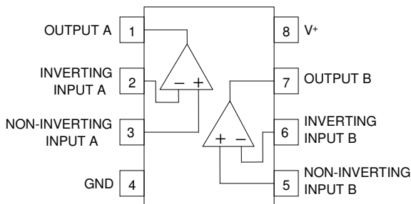
S.O package8
