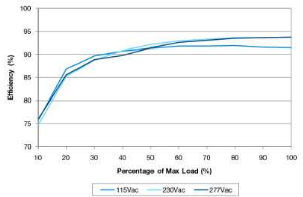
LNE-48V185W□
