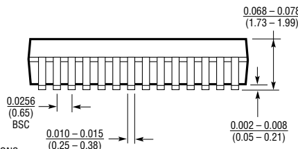
28SSOP 0894
