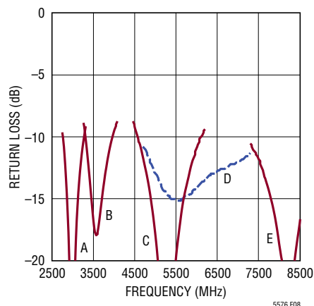
Figure 8. OUT Port Return Loss Tuned for (A) 3000MHz, (B) 3500MHz, (C) 5200MHz, (D) 5800MHz, (E) 8000MHz
