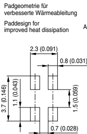
Fläche darf bei Verwendung von TOPLED® elektrisch nicht beschaltet werden. For TOPLED® assembly do not use this area for electrical contact
