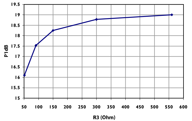
P1dB
