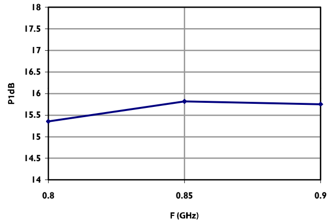
P1dB
