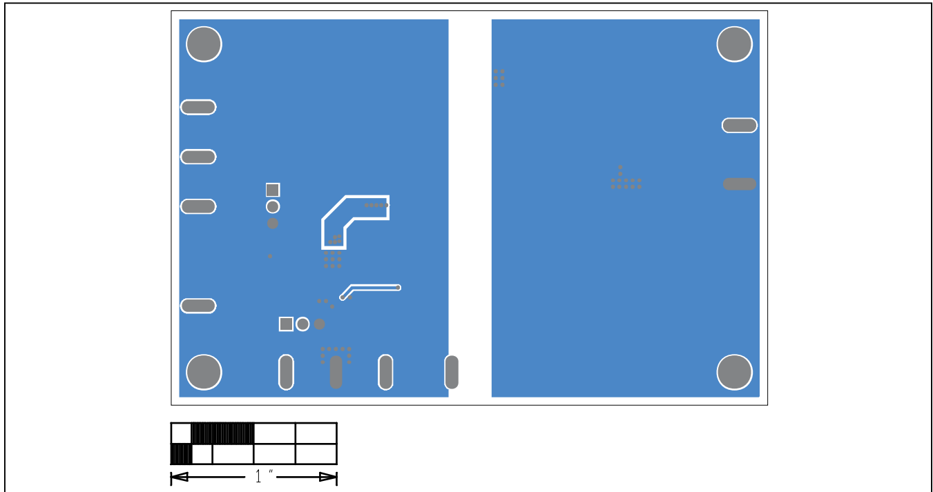
MAX17682EV—Bottom
