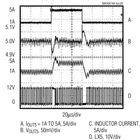
OUT5 LOAD TRANSIENT
