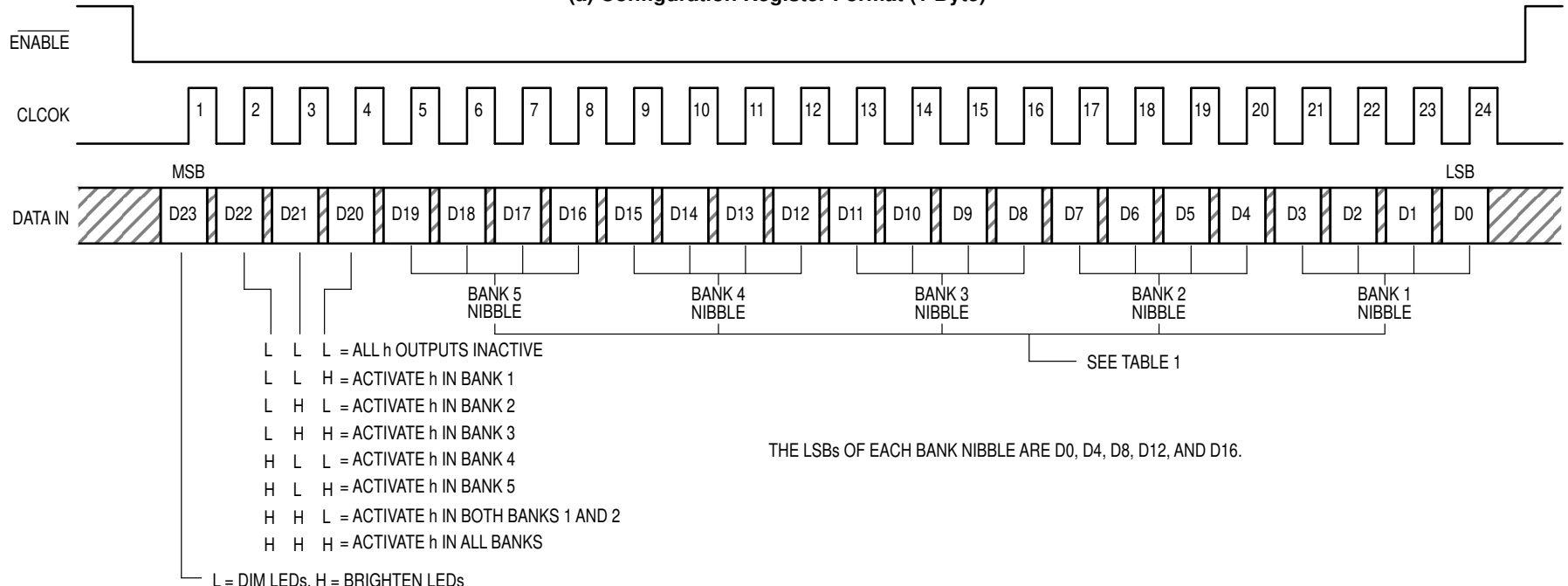
(b) Display Register Format (3 Bytes)
