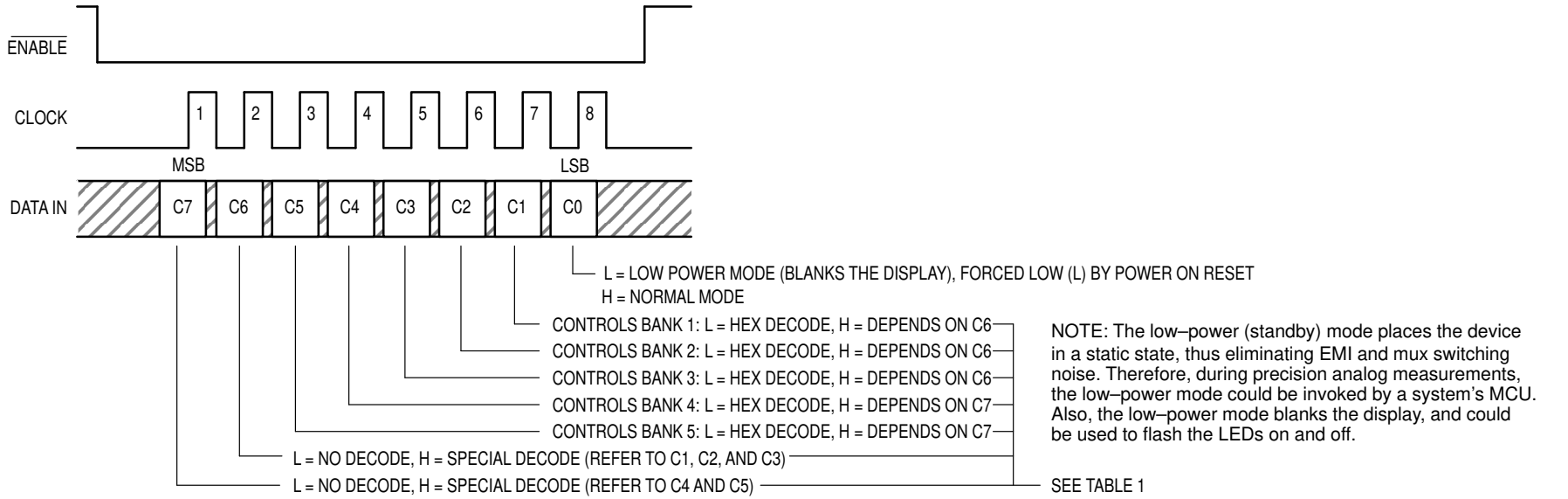
(a) Configuration Register Format (1 Byte)
