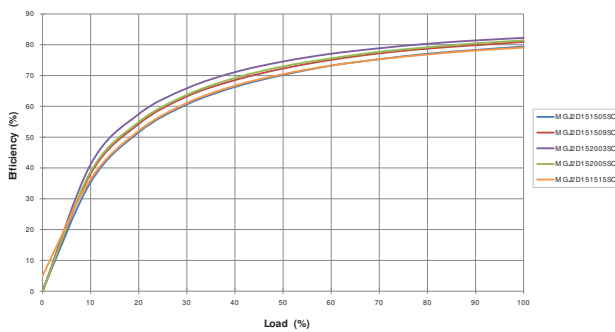
15V INPUT
