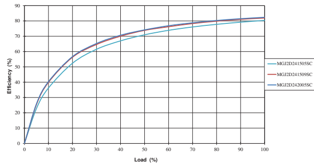
24V INPUT
