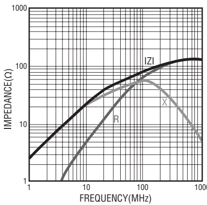
MH 4516- 800Y
