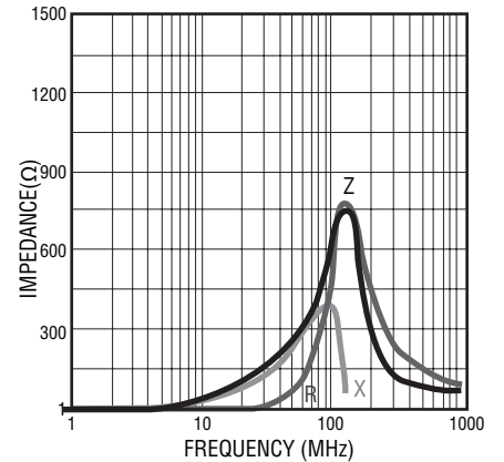
MH 4516- 750Y
