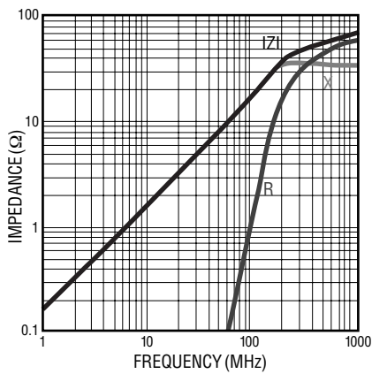
MH 3261- 190Y
