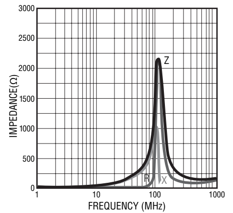
MH 4516- 102Y
