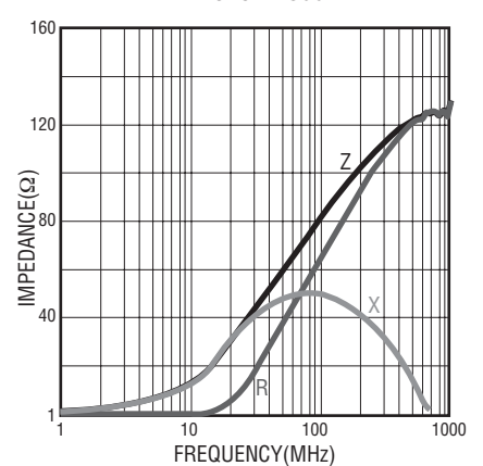
MH 3261- 800Y
