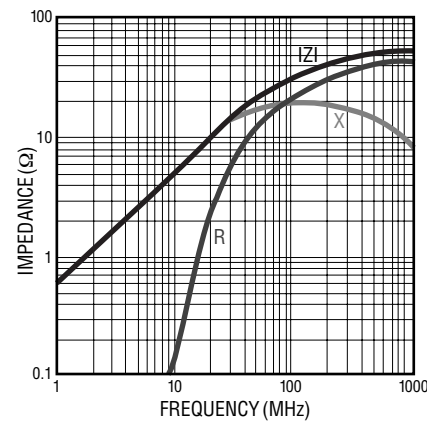
MH 3261- 310Y
