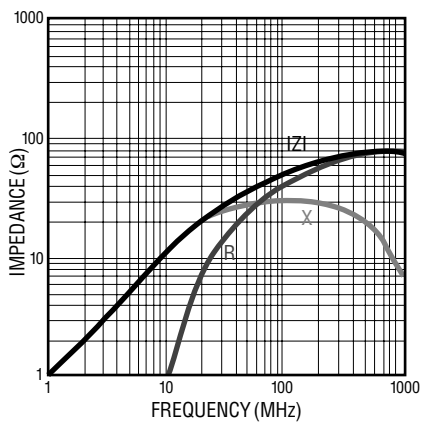
MH 3261- 500Y
