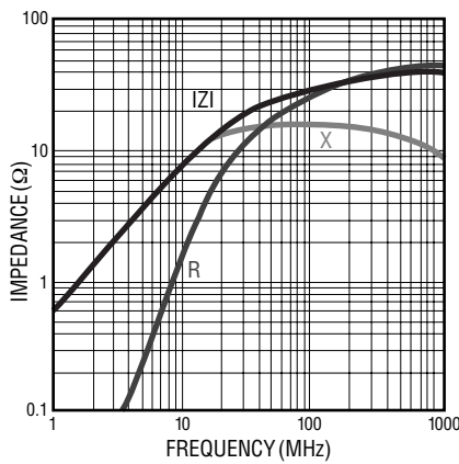
MH 3261- 260Y
