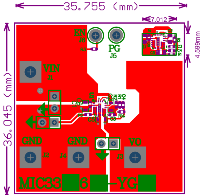
Top
