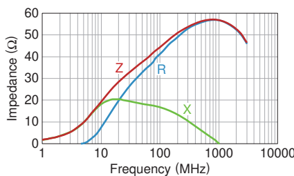
MMZ2012S400ATD25
