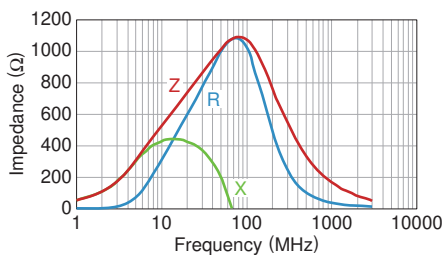
MMZ2012R102ATD25
