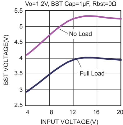
BST vs. Vin
