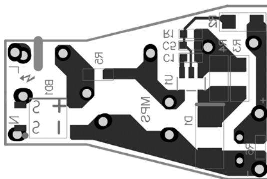
Bottom Layer
