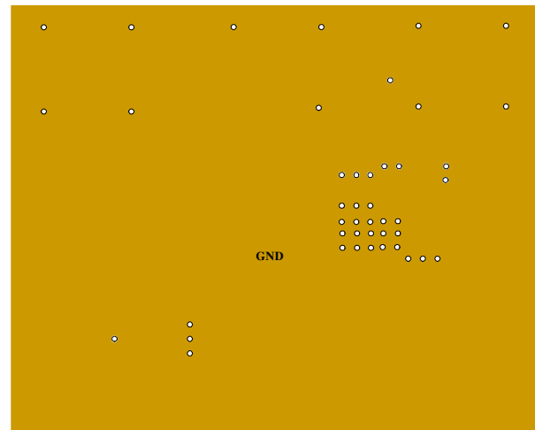
Inner1 Layer
