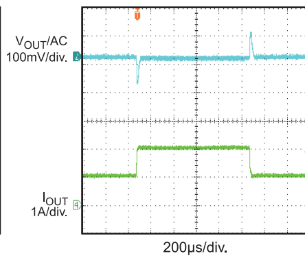
Load Transient I_{OUT}=1A \leftrightarrow 2A , 1.6A/\mu s
