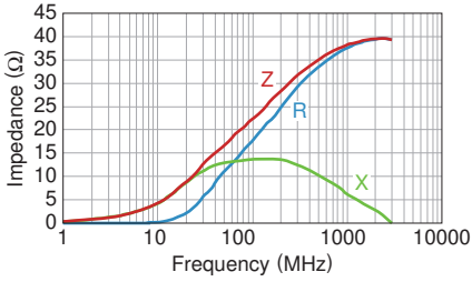
MPZ0603S220CT000
