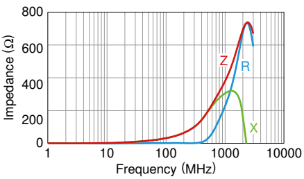
MPZ1005F330ETD25
