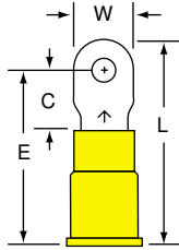
MV10-4R/S 4 12-10
