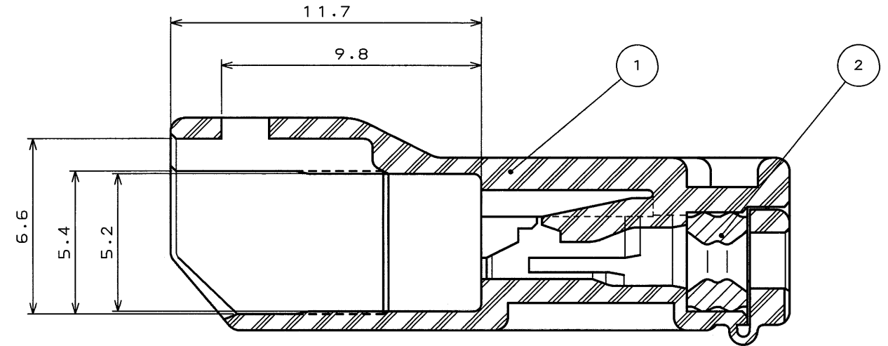
SECT. A-A (SCALE 5:1)
