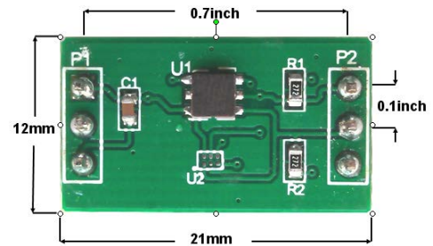
MXC6226XU-B
