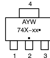
SOT-223 ST SUFFIX CASE 318E
