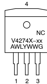
D2PAK DS SUFFIX CASE 418AF
