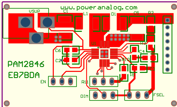
Top Layer
