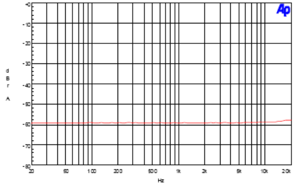
17. CMRR
