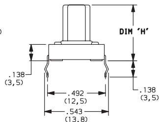
PTS125SM12 SPST
