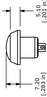
DOMED ACTUATOR
