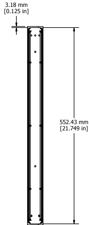
SECTION A-A
