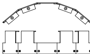
前红外安装支架 front IR mounting bracket
