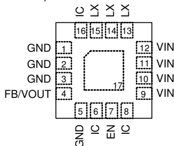
WQFN-16L 3x3 (RT8010A)
