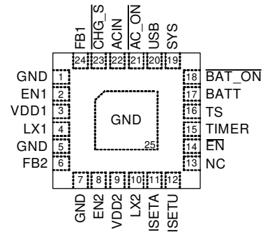
WQFN-24L 4x4
