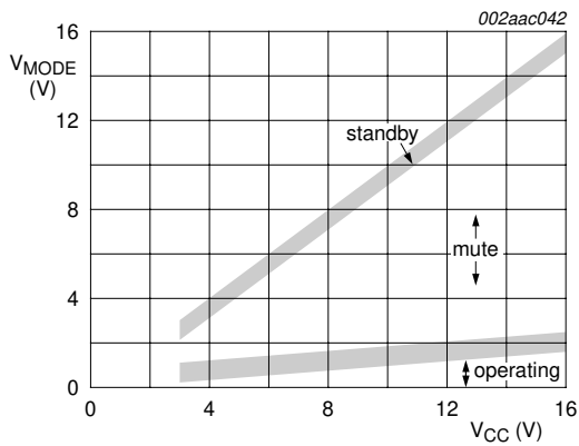
Fig 6. V_{MODE} versus V_{CC}
