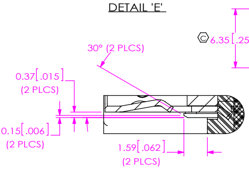
SCALE 4:1
