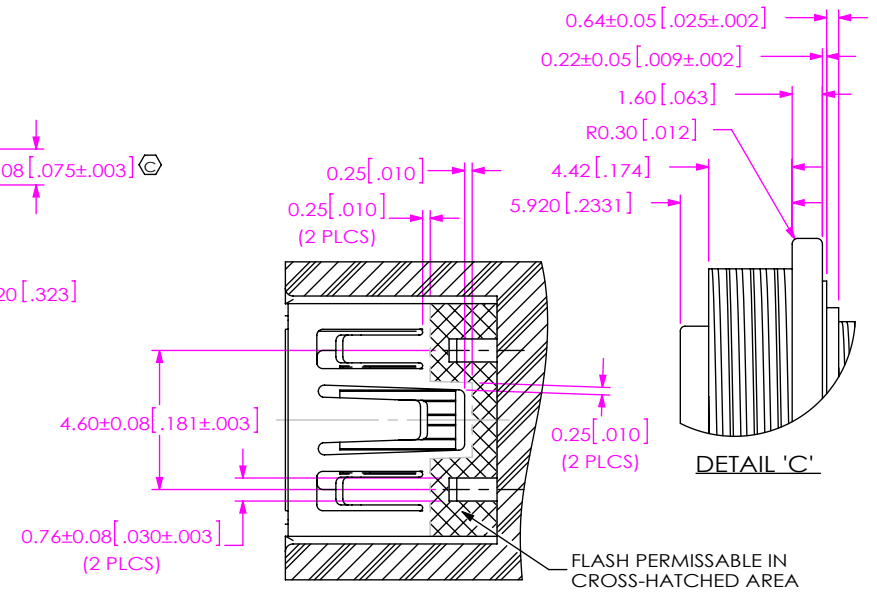
SCALE 4:1
