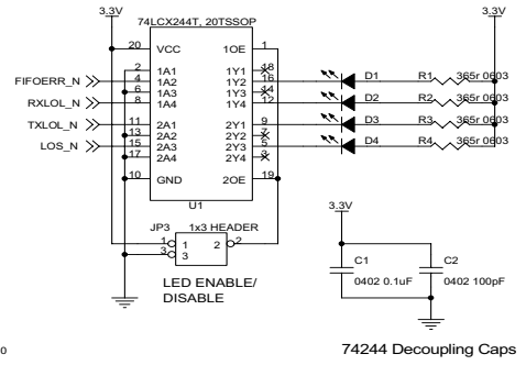
74244 Decoupling Caps
