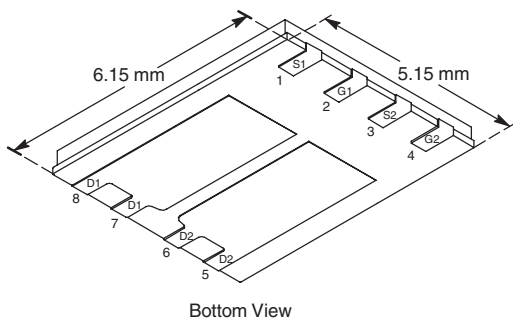
PowerPAK SO-8
