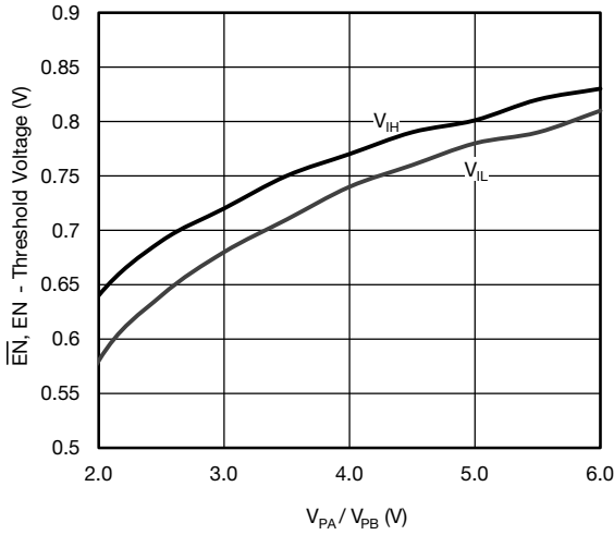
Fig. 15 - EN Threshold Voltage vs. Input Voltage
