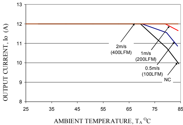
V_o=3.3V
