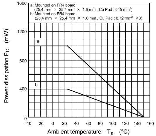
Fig. 7.14 P_D - T_a
