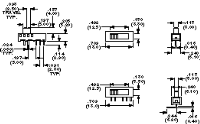
P. O. HOLE LAYOUT
